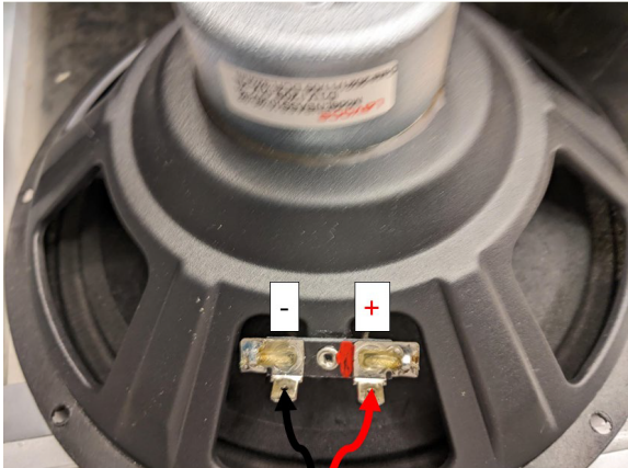
Wire 1/2
